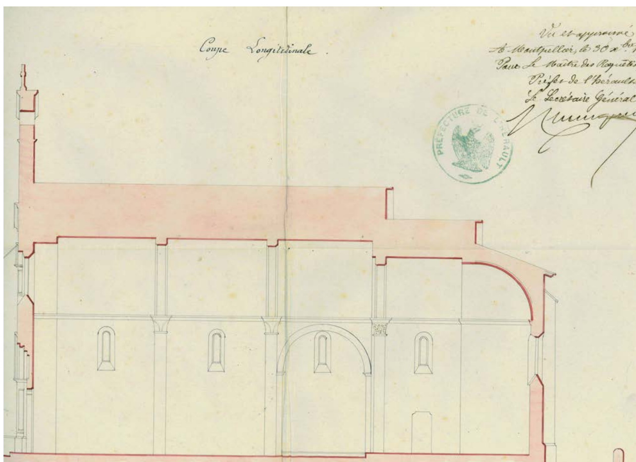
2M1 – Dessin de l'église (1856)
