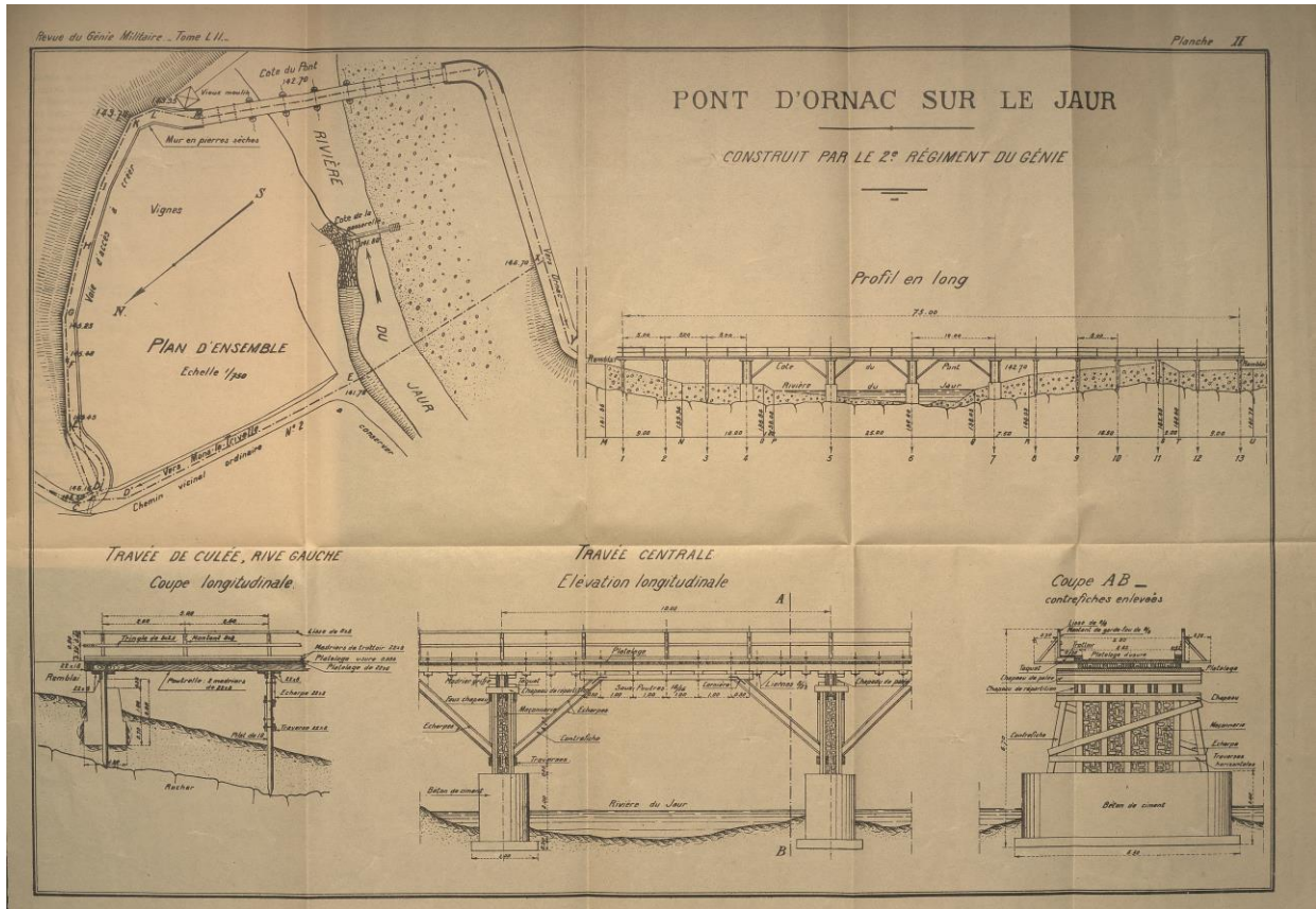
1010 — "LE PONT D'ORNAC SUR LE JAUR CONSTRUIT PAR LE 2 EME REGIMENT DU GENIE" (1923)
