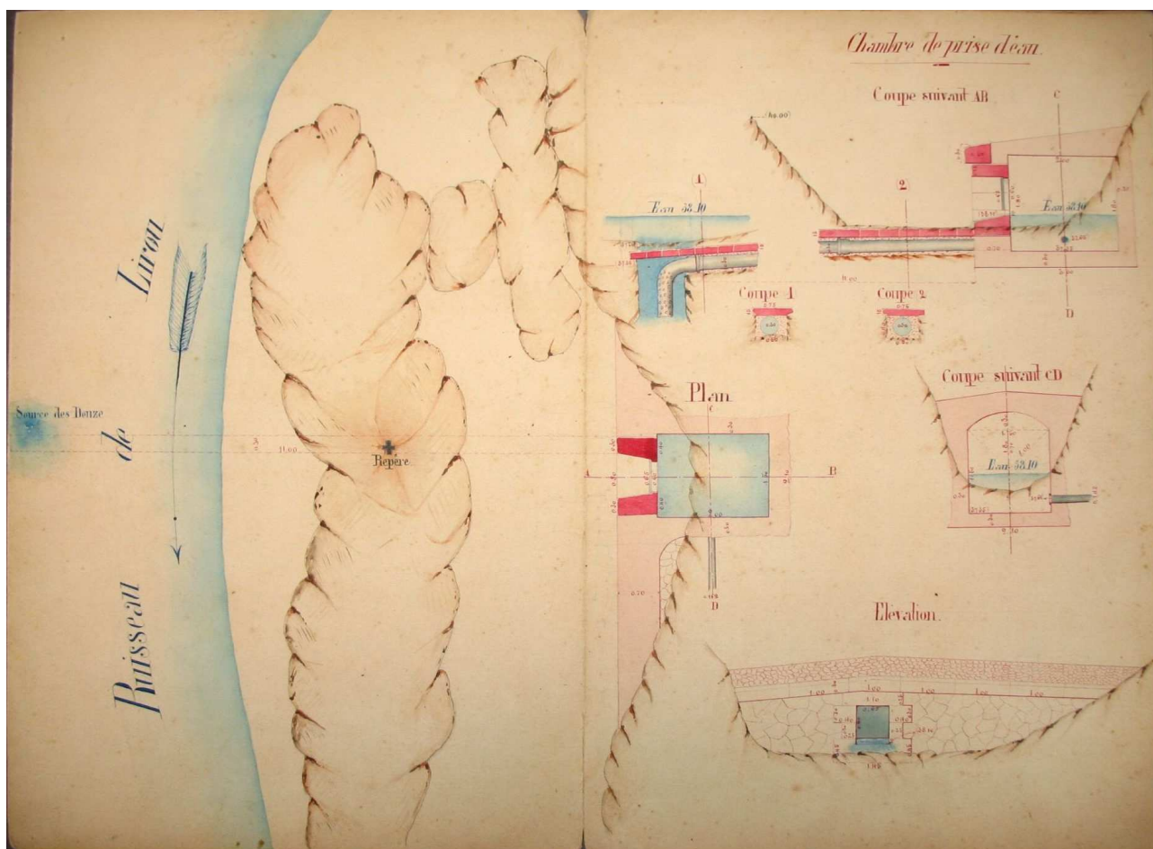
1039 - Plan de l'avant-projet de distribution des eaux de la source de la Douze (1878).
