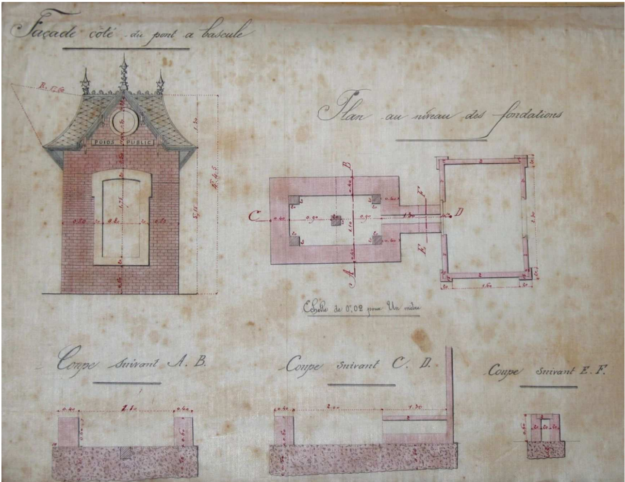
1M7 - Plan du pont à bascule (1879).
